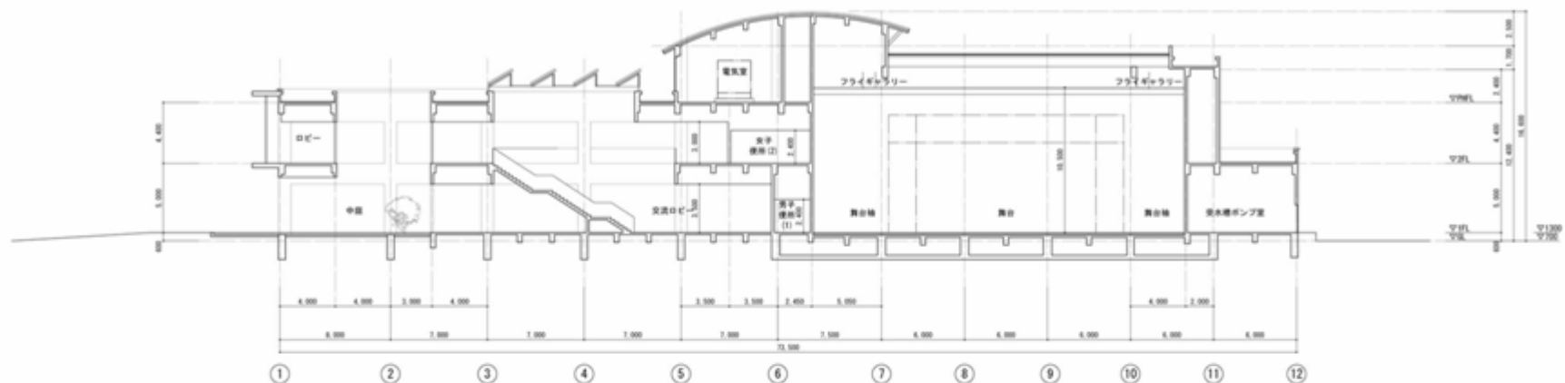
A-A断面図
