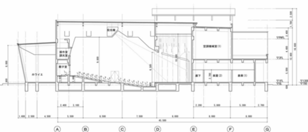
B-B断面図
