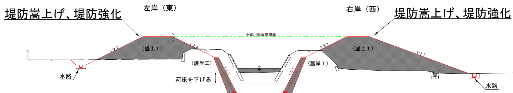
末政川 整備断面（有井橋から上流）
