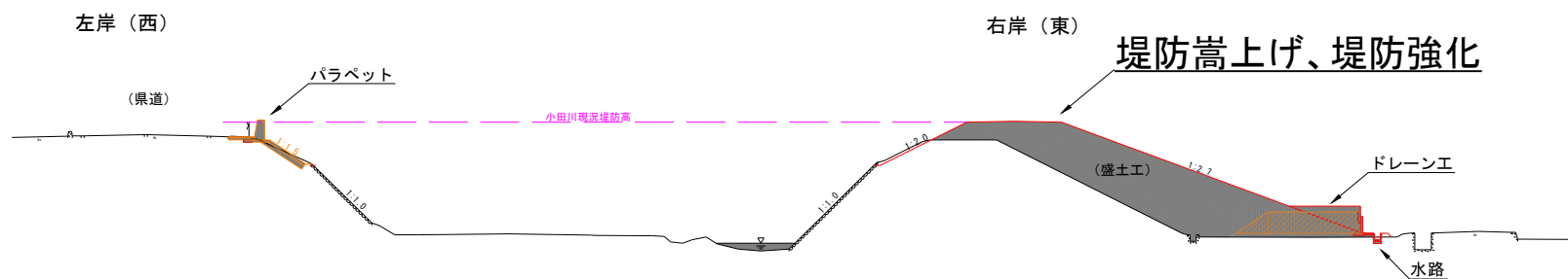
真谷川 整備断面（県道沿い区間）
