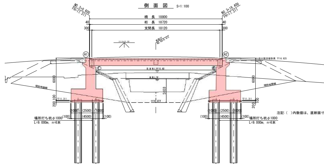
(2) 側面図
