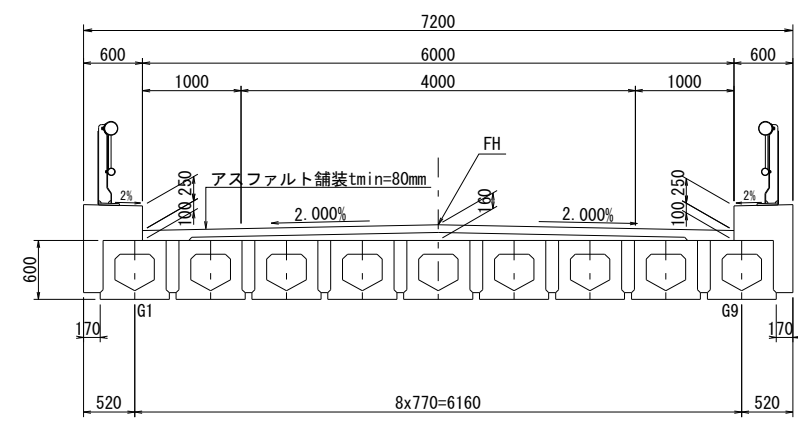
(3) 上部断面図
