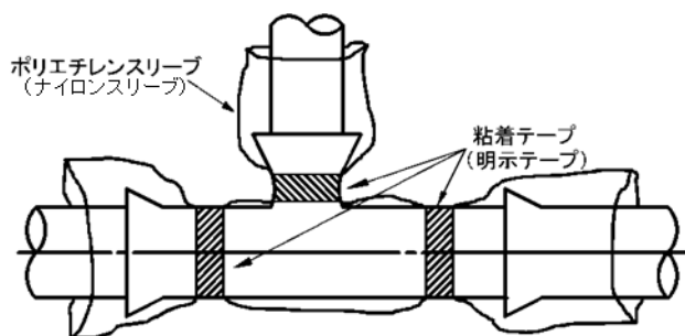
図 2-1 防食用ポリエチレンスリーブ被覆及びナイロンスリーブ被覆
