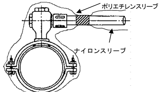
図 2-1 防食用ポリエチレンスリーブ被覆及びナイロンスリーブ被覆
