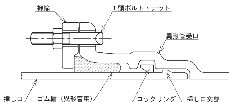
図2-8 GX形管（異形管受口）の接合
