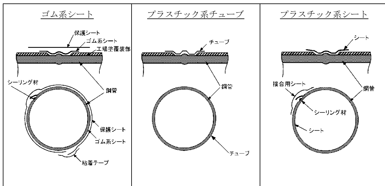
図2-7 ジョイントコートの巻付け
