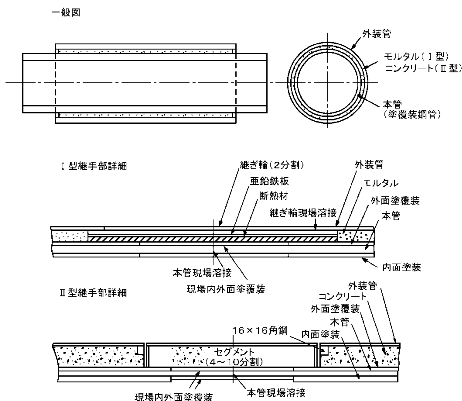
図 2－17 水道用推進鋼管
