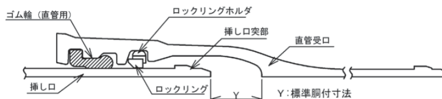
図2-7 GX形管（直管）の接合
