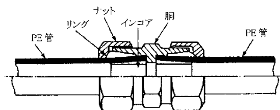
図 2－1 1 水道用ポリエチレン管金属継手（JWWA B 116）の接合方法
