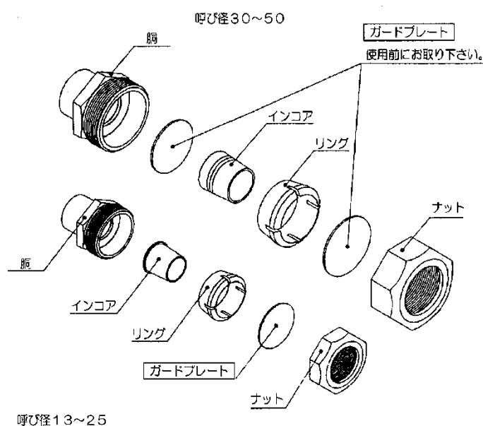
図 2－1 2 水道用ポリエチレン管金属継手（JWWA B 116）の各部品名称
