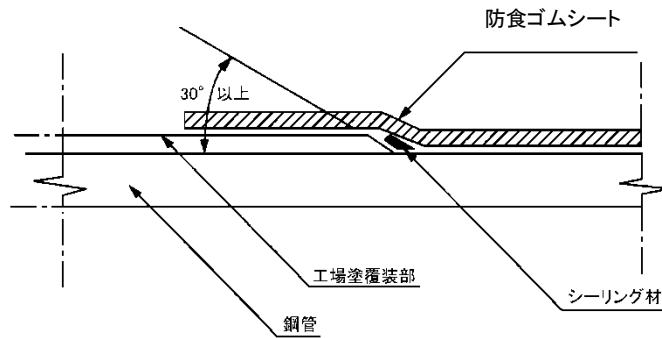
図 2-8 シーリング材の施工
