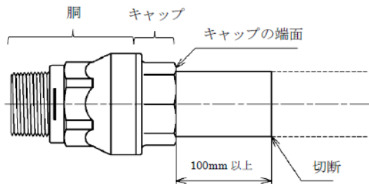
図 2-15 管の切断
