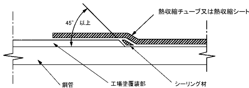
図 2-9 シーリング材の施工
