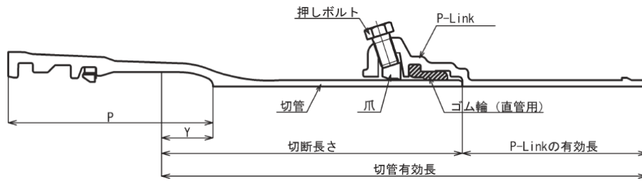
図2－9 GX形管（P - Link）の接合
