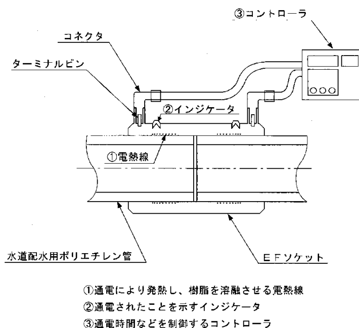
図 2－10 E F 接合
