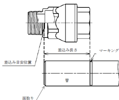
図 2－１３ 差し込み長さ
