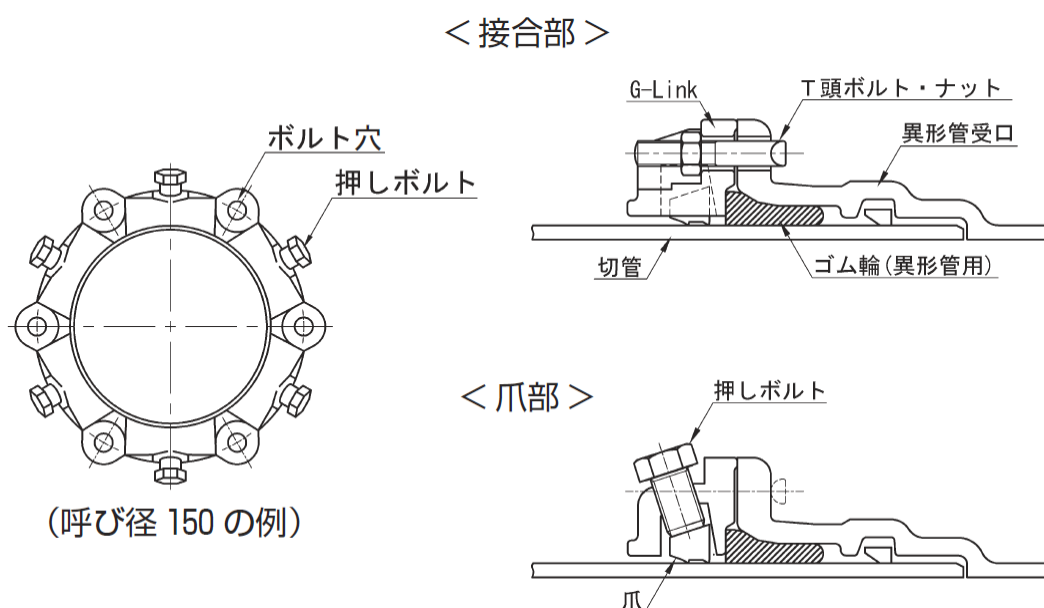
図2-10 GX形管（G - Link）の接合
