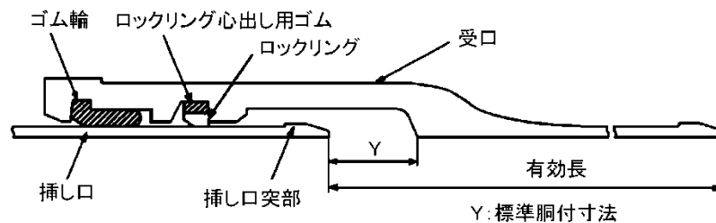
図 2-5 NS形管（直管）の接合
