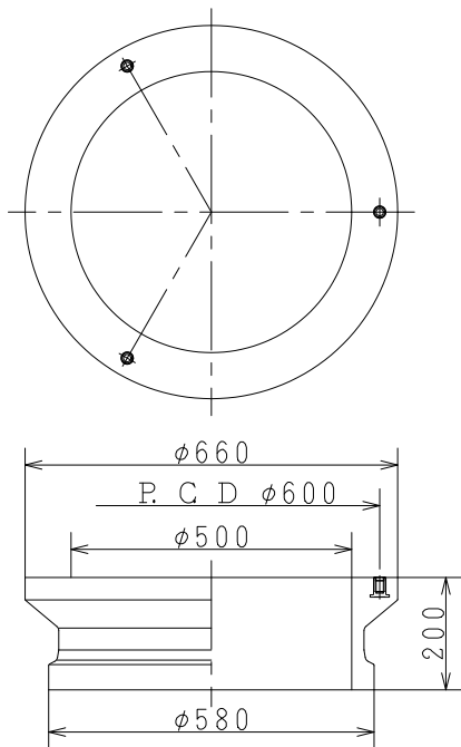
倉敷市型円形3号200A (円形3号RB50(A))
