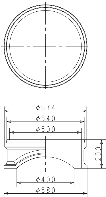
倉敷市型円形3号200CTK (円形3号RB50(CTK))
