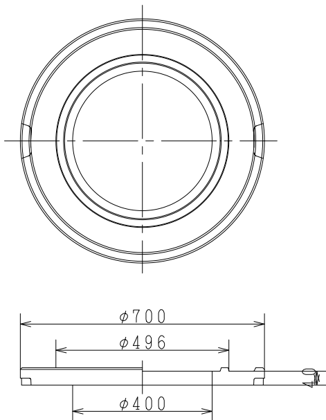
倉敷市型円形3号40P (円形3号RB50(P))
