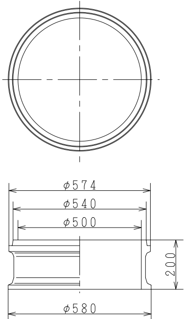
倉敷市型円形3号200C (円形3号RB50(C))
