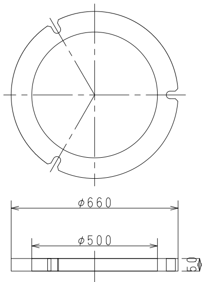
倉敷市型円形3号50K (円形3号RB50(K))
