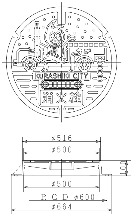
倉敷市型円形3号鉄蓋 (円形3号(500))
