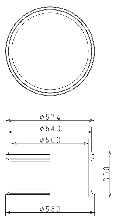
倉敷市型円形3号40PTK (円形3号RB50(PTK))
