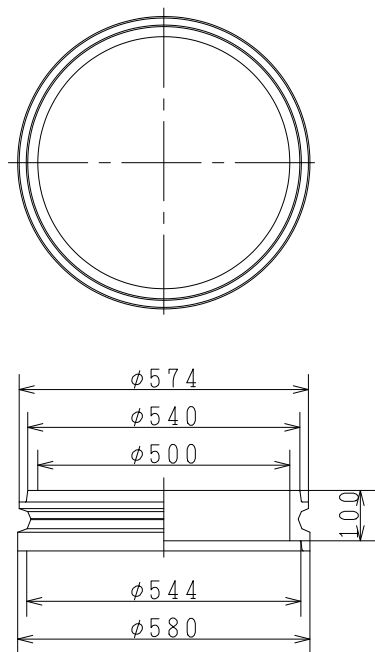
倉敷市型円形3号100B (円形3号RB50(B))
