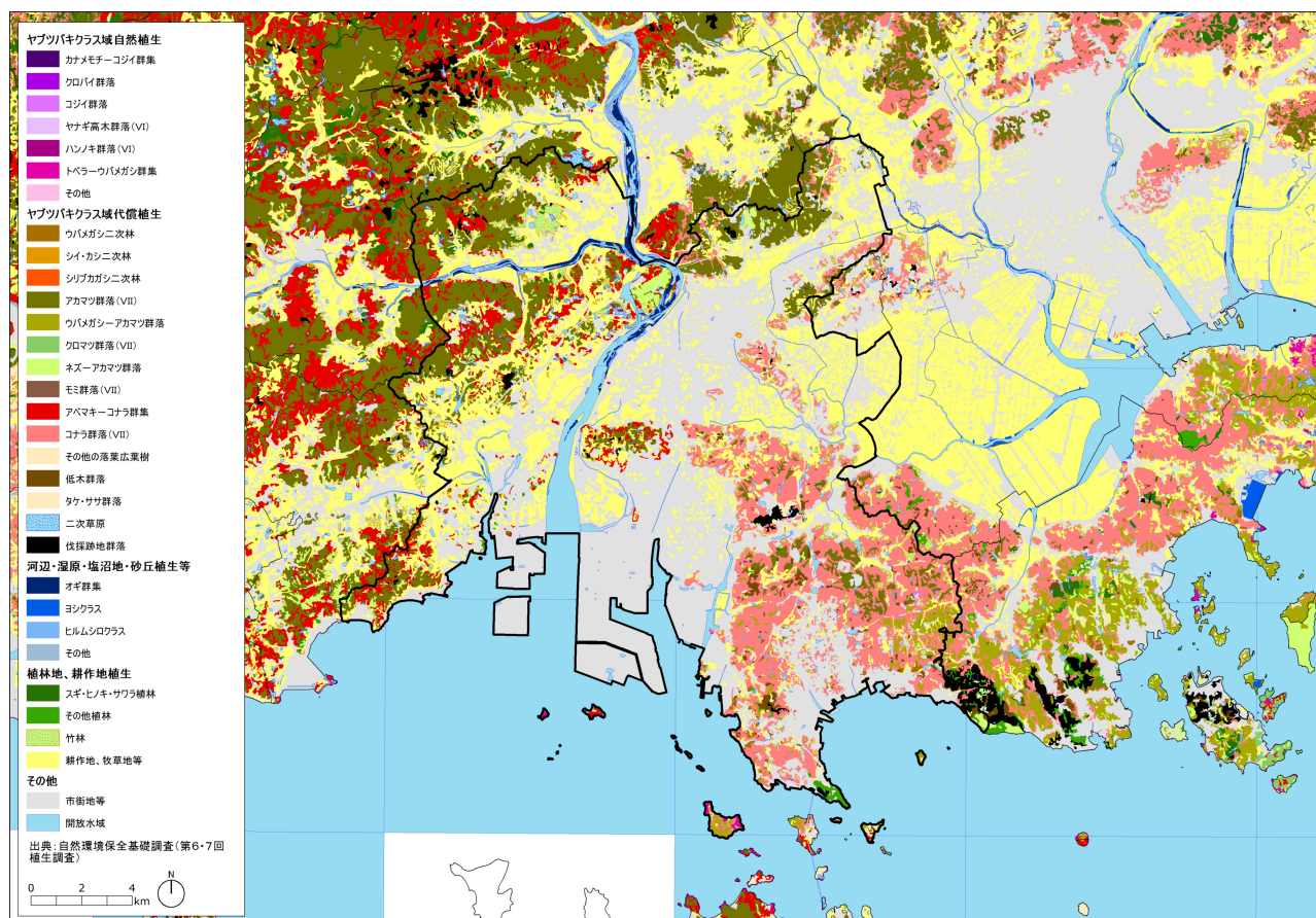
図 2－5 植生図
