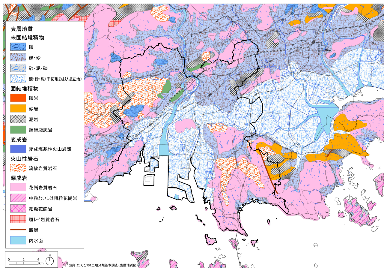
図 2－3 表層地質図
