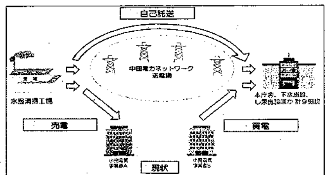
倉敷市における自己託送のイメージ
