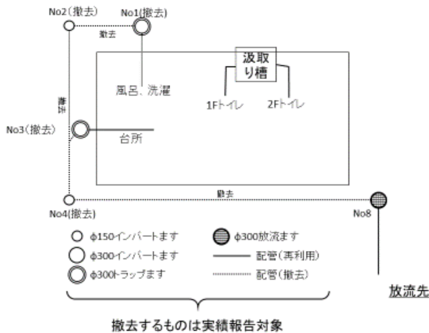
既存排水経路図（汲取り槽）
