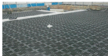
▲事業者によるプラスチック貯留槽の設置
