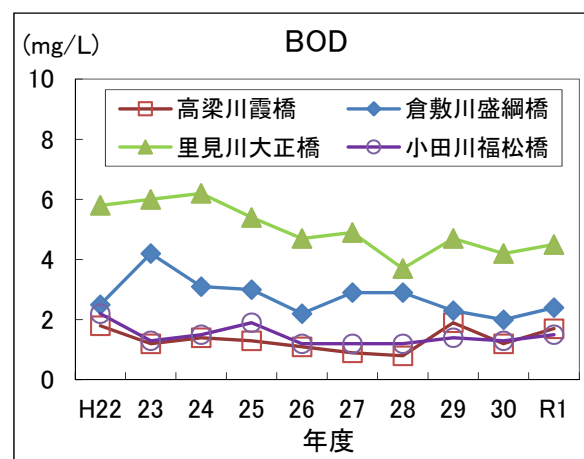
市内河川におけるBODの経年変化(75%値)
