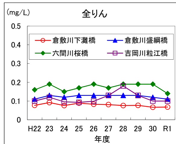
倉敷川4測定点における全窒素及び全りん*の経年変化(年平均値)
