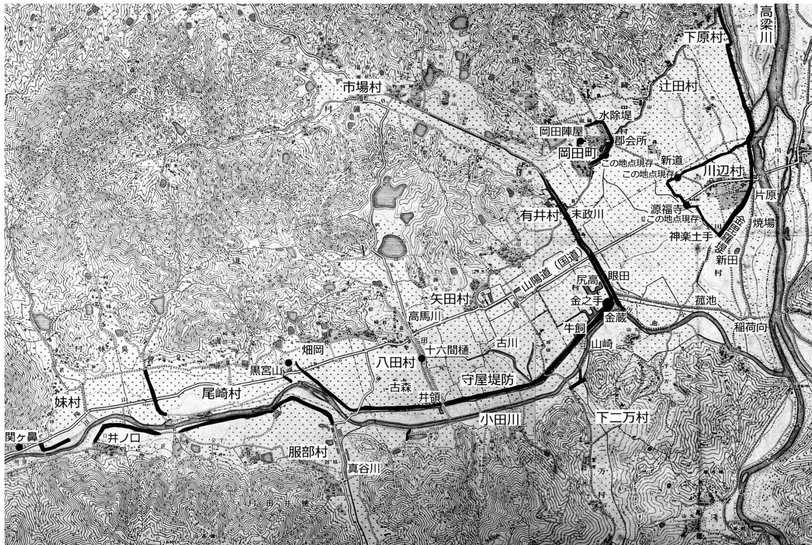
図2 宝永元年（1704）守屋勘兵衛重行による新堤防建造・川筋付替え後の小田川下流域
