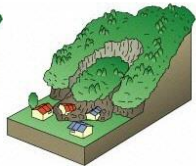
地滑り
